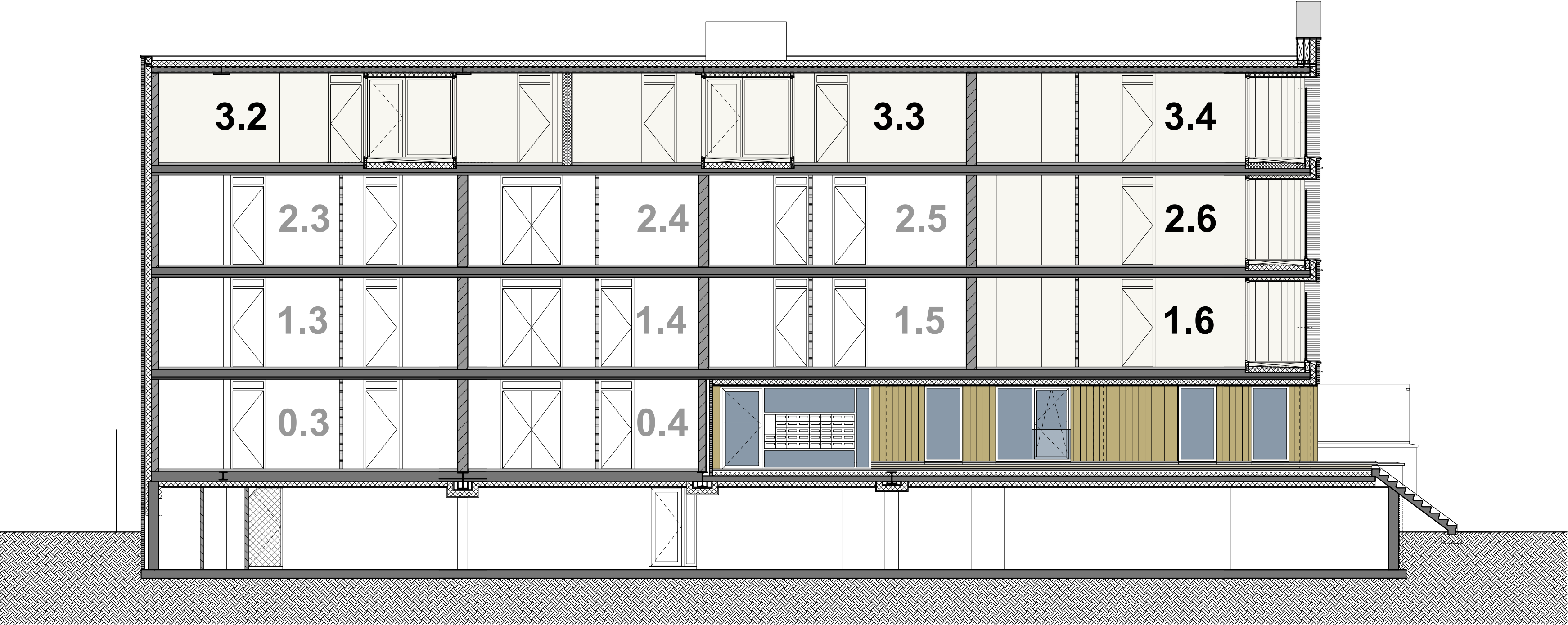
doorsnede CC
