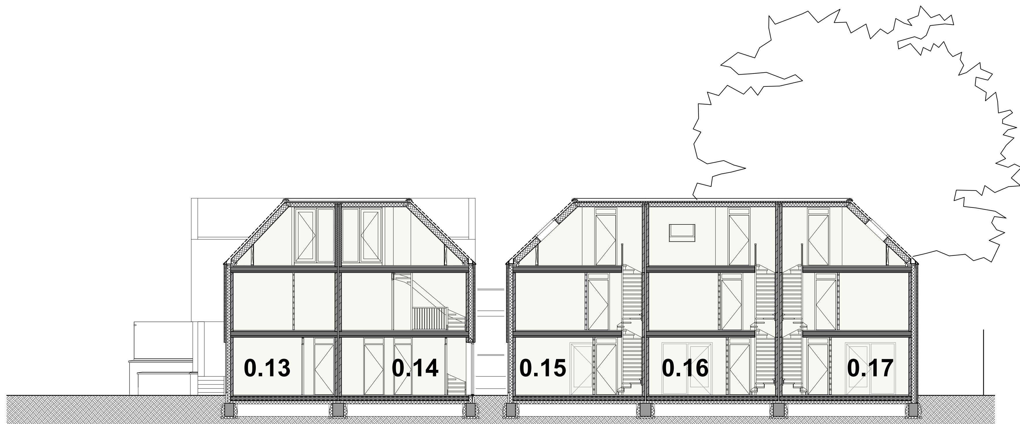
doorsnede BB
