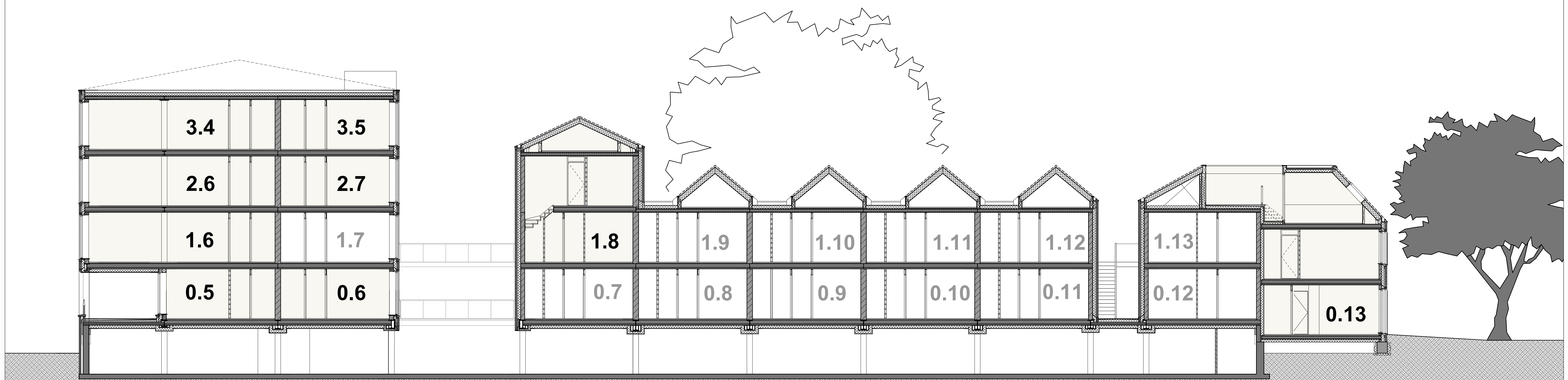
doorsnede AA
