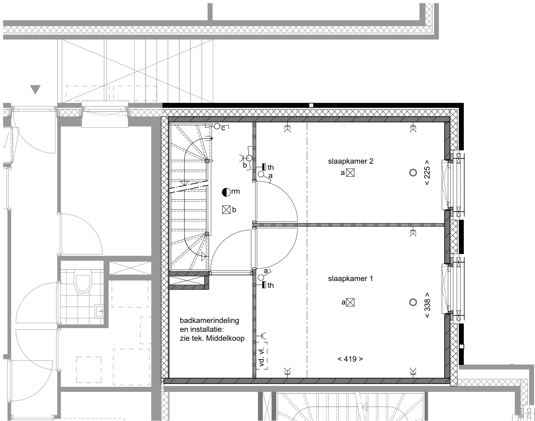
eerste verdieping
