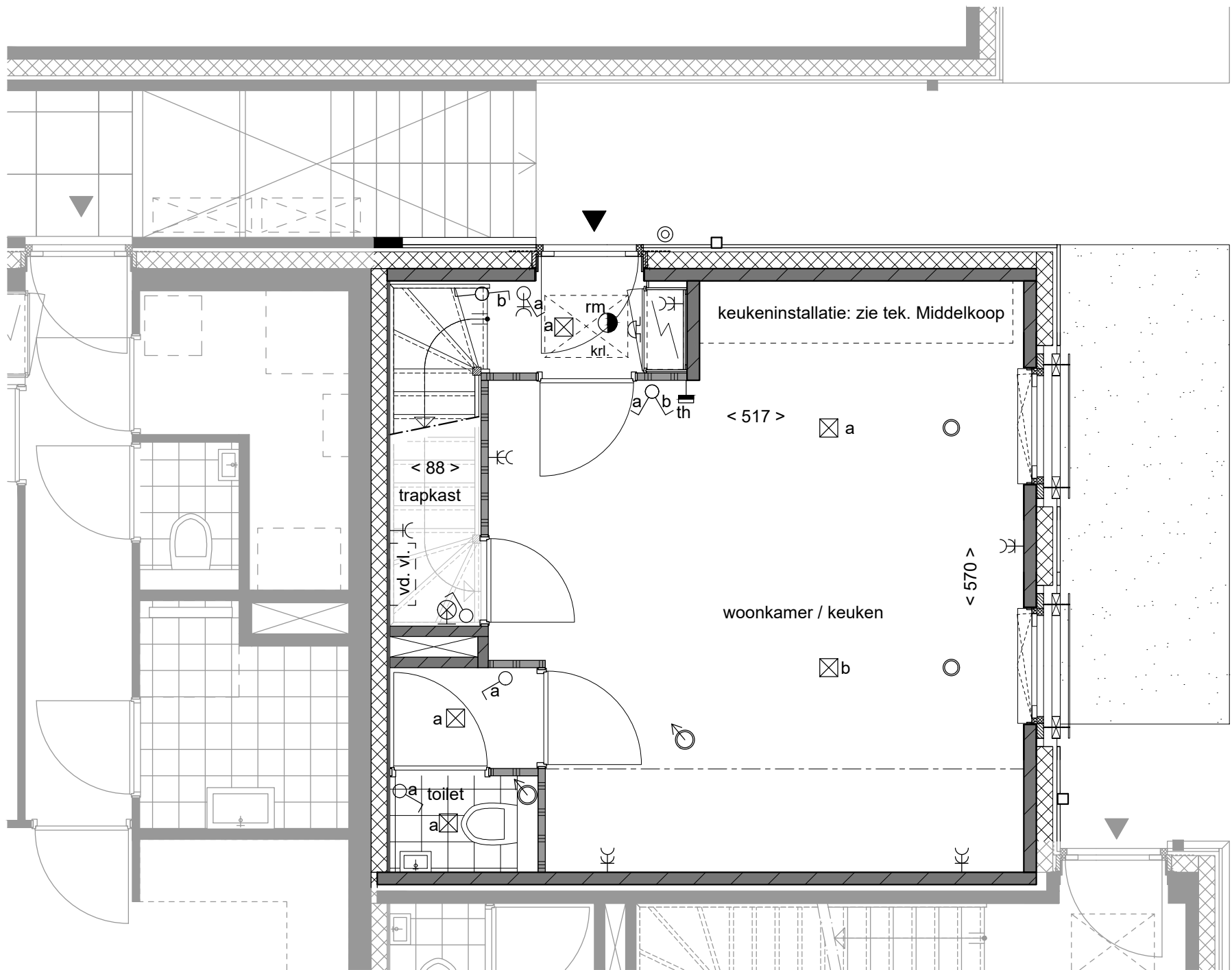
begane grond
