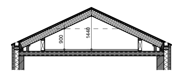
doorsnede A schaal 1:100
