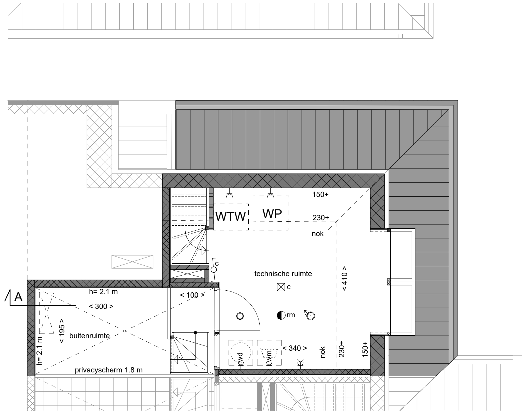
tweede verdieping
