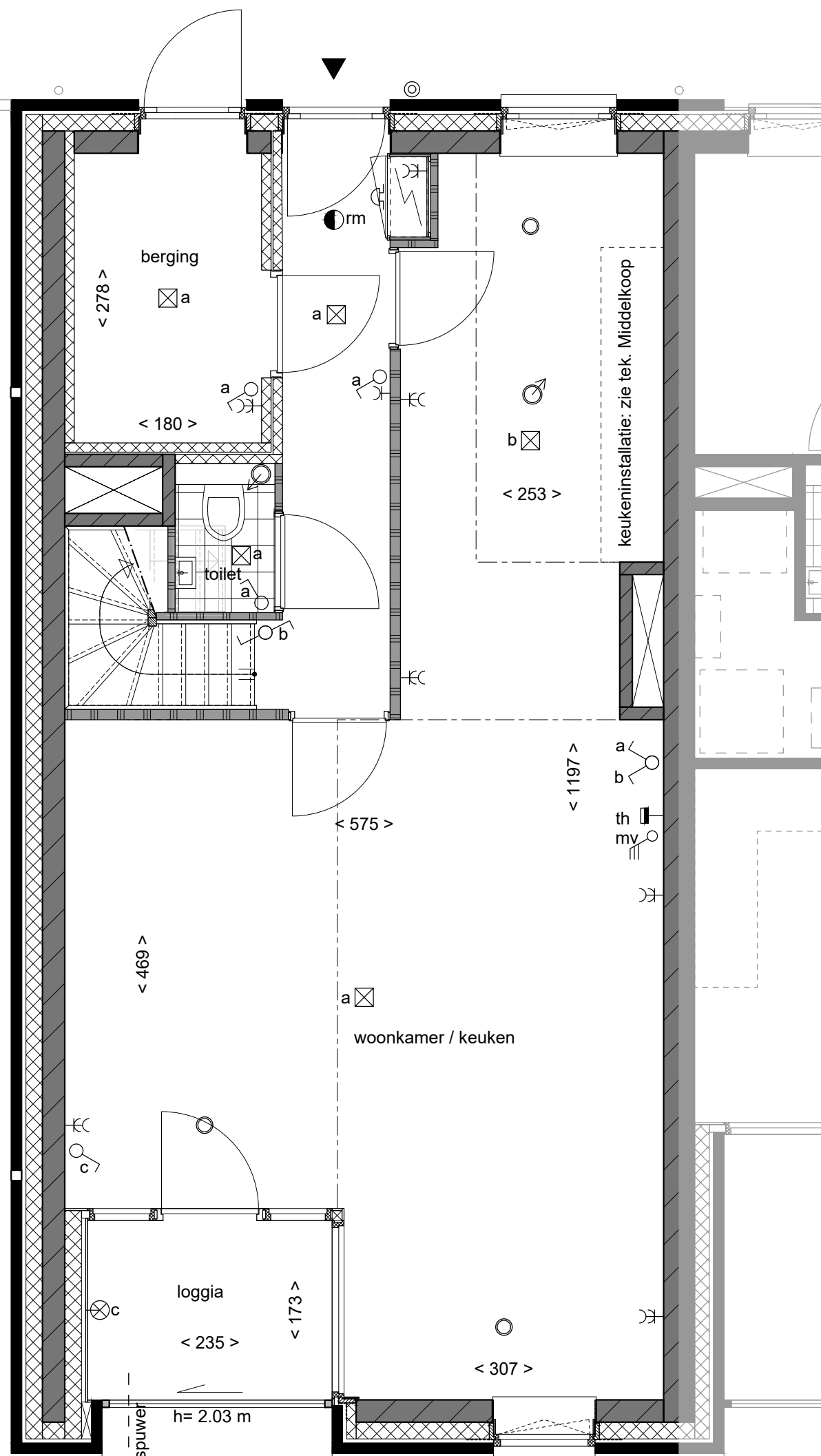
eerste verdieping
