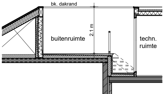
doorsnede A schaal 1:100
