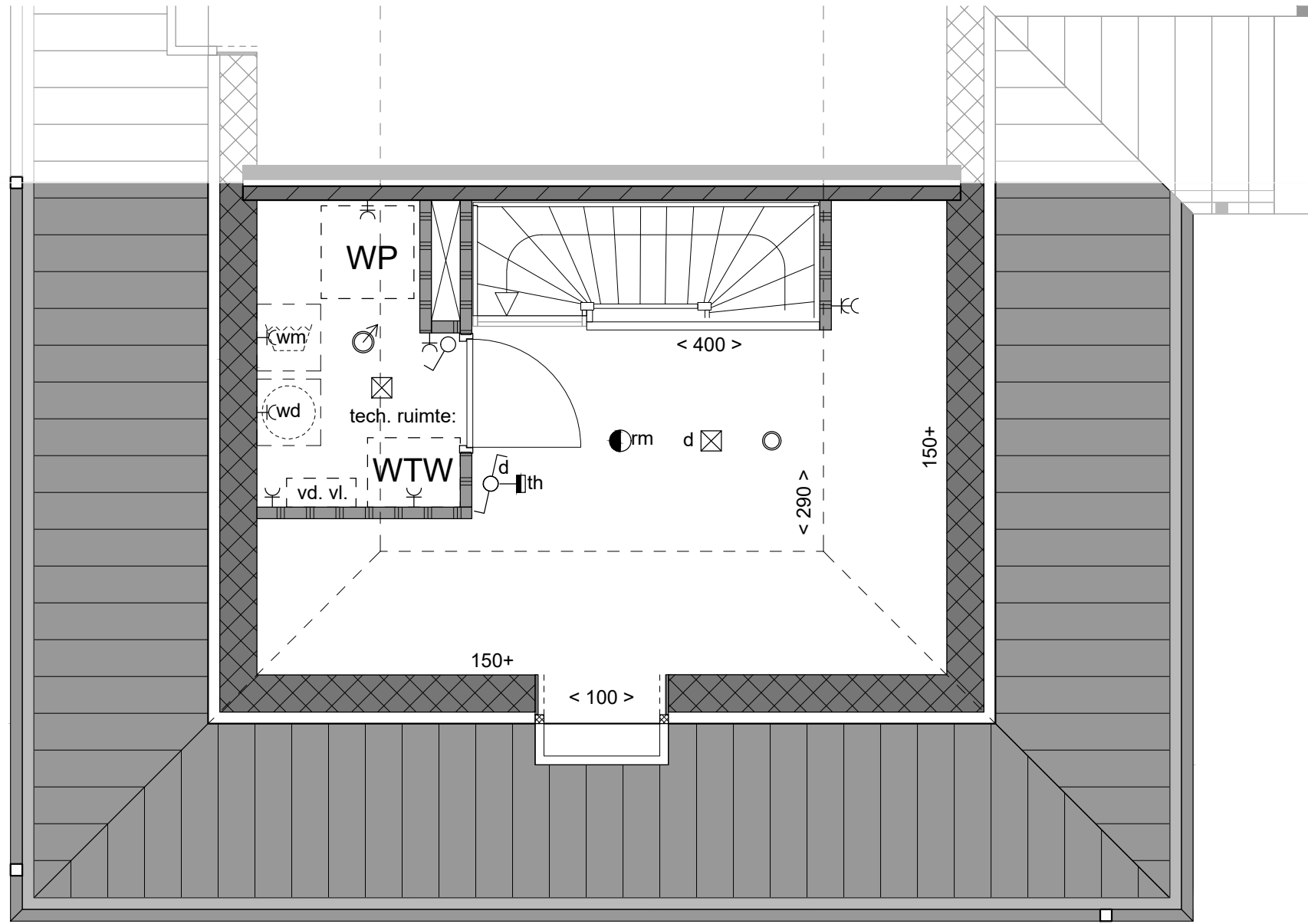
tweede verdieping
