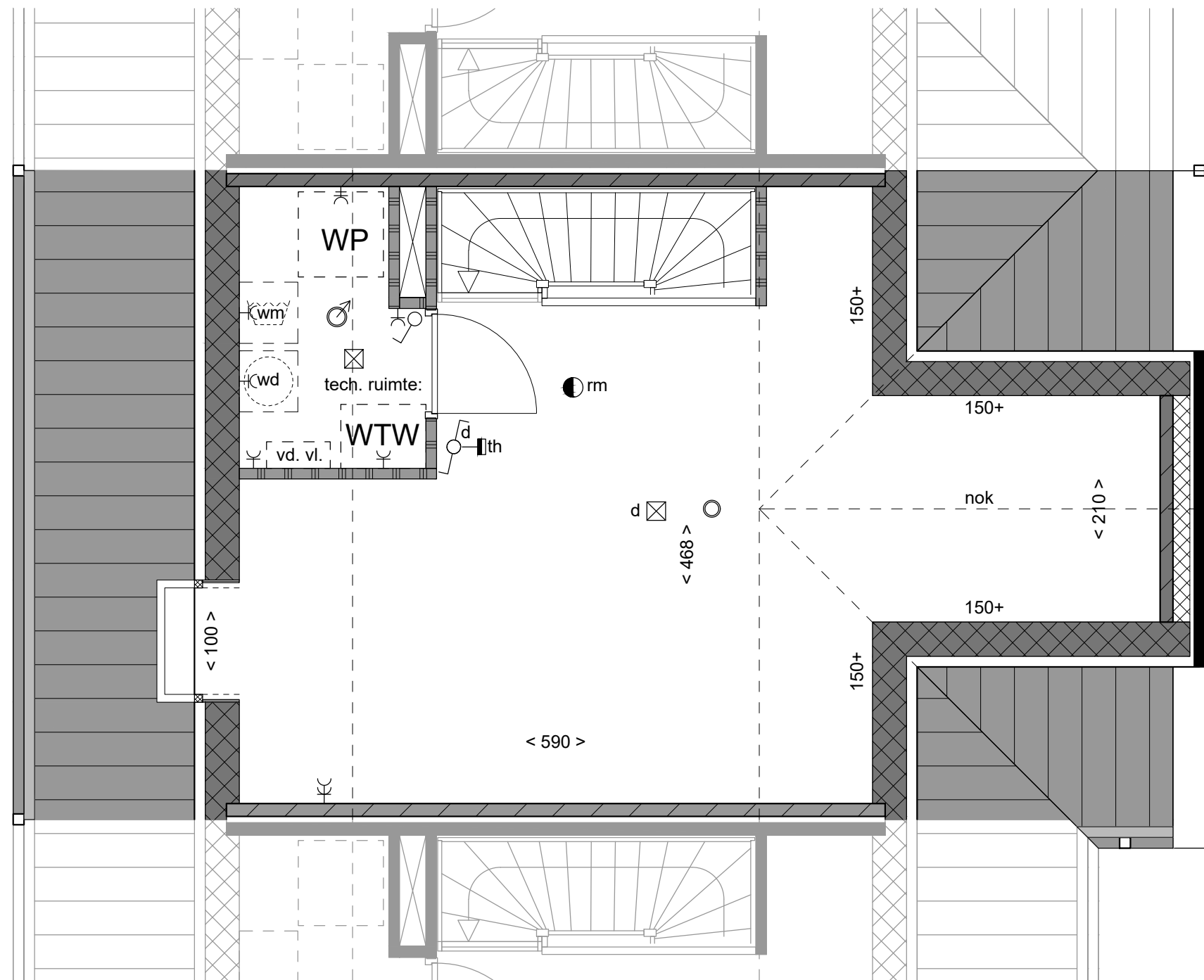
tweede verdieping
