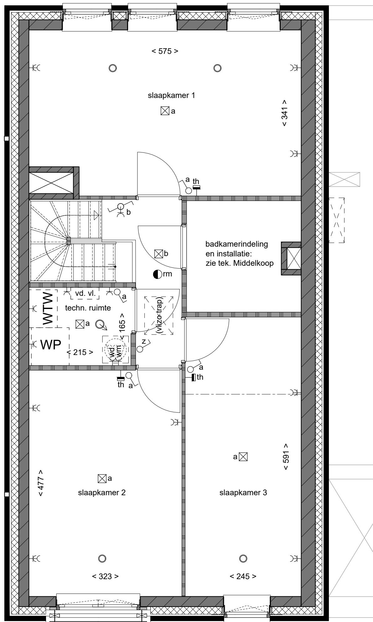
tweede verdieping
