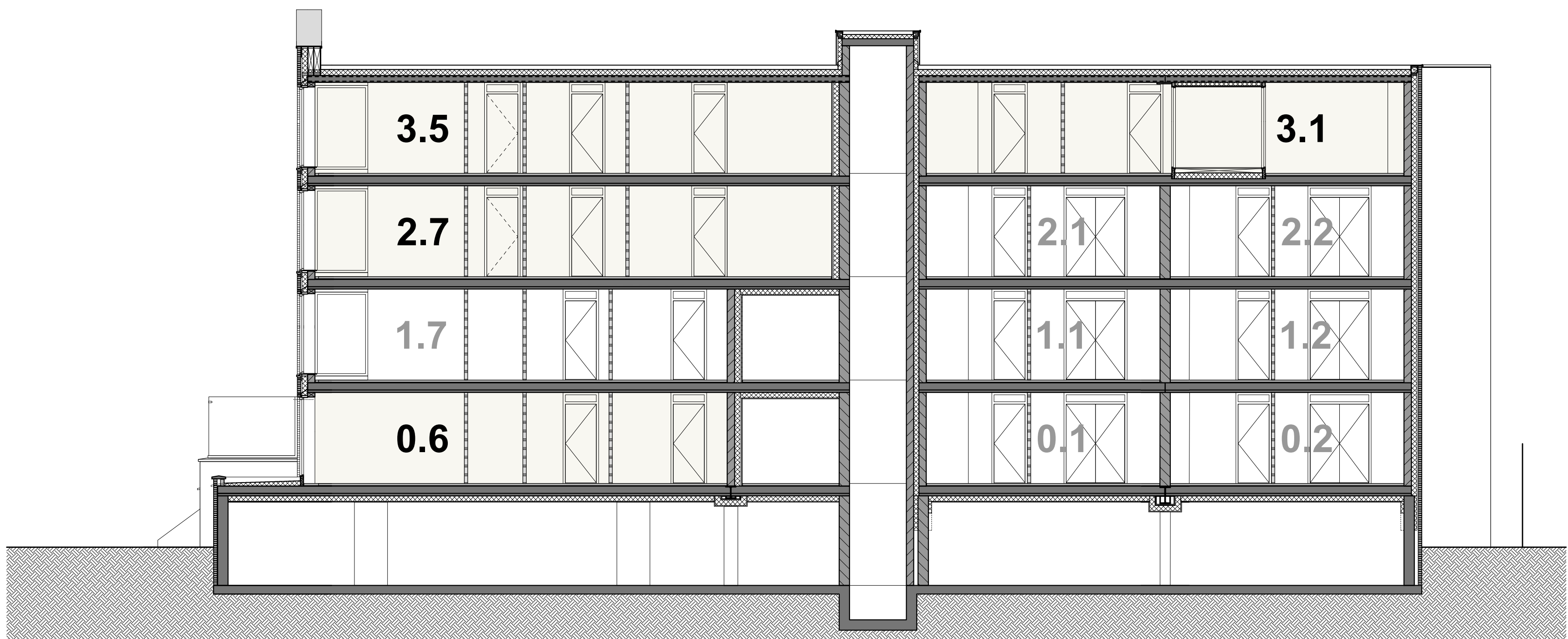
doorsnede DD
